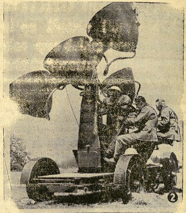
En la fotografía puede verse un localizador de sonido y los hombres que lo manejan. Los cuatro tambores son mecanismos auditivos de gran sensibilidad que cogen el sonido de los aviones que se aproximan, lo registran automáticamente dan su altura, dirección y la distancia a que se encuentran, para servir de guía a los artilleros antiaéreos.
